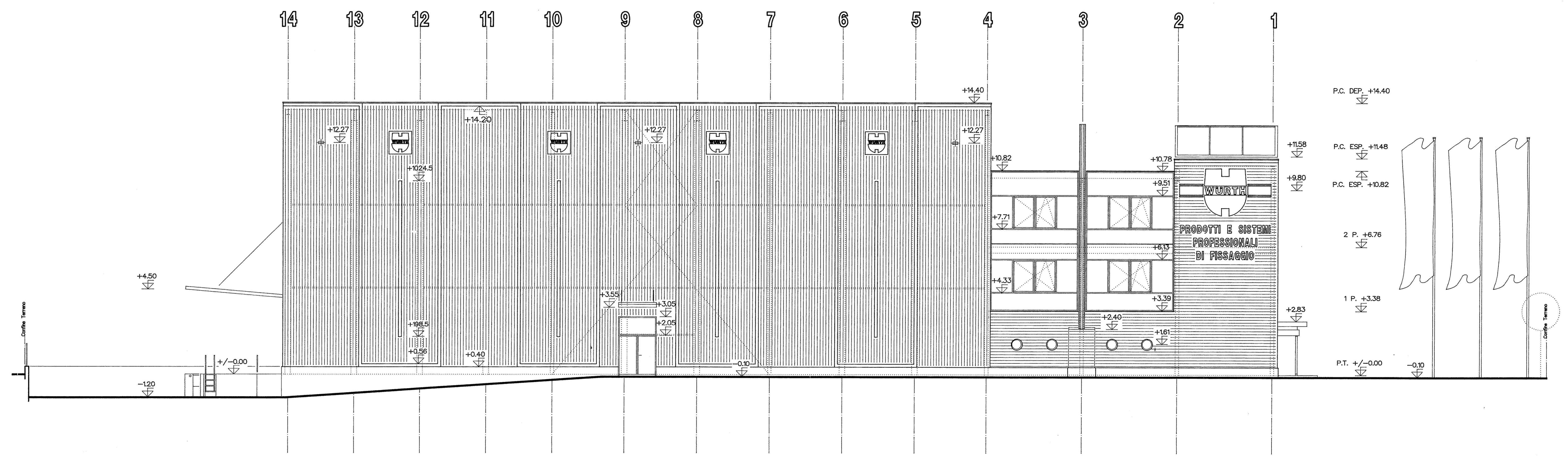
FACCIATA EST
