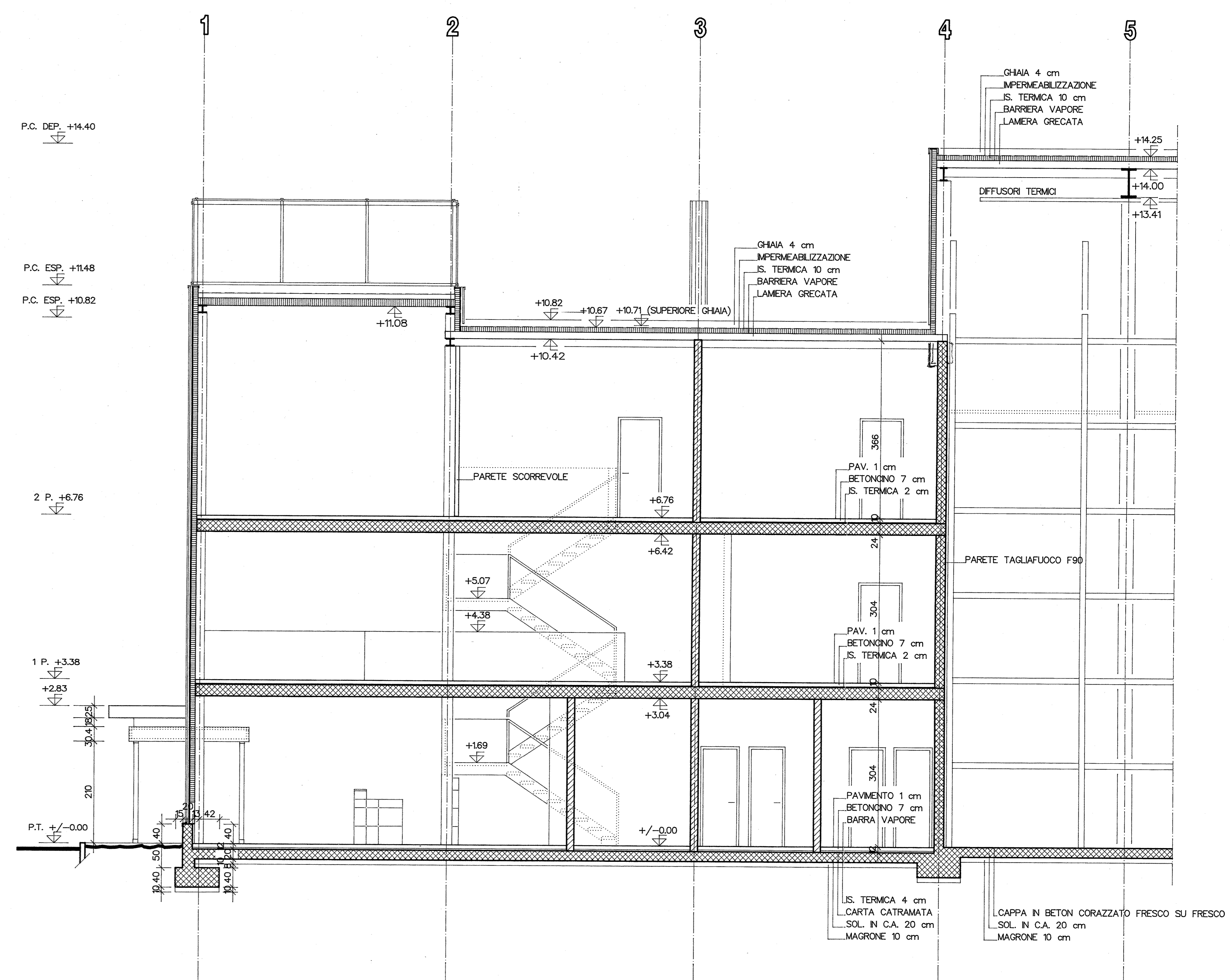
SEZIONE C-C
