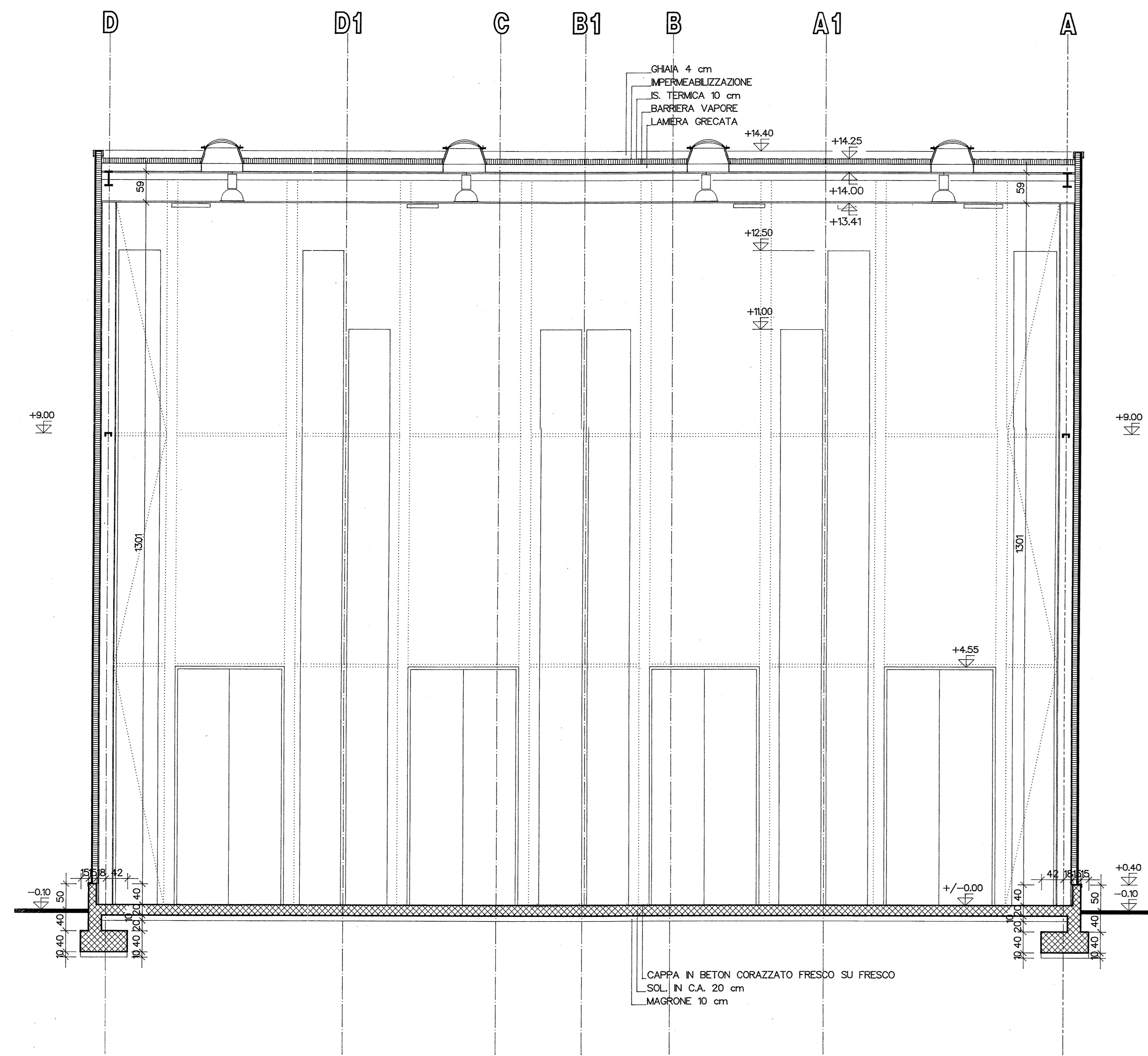
SEZIONE B-B
