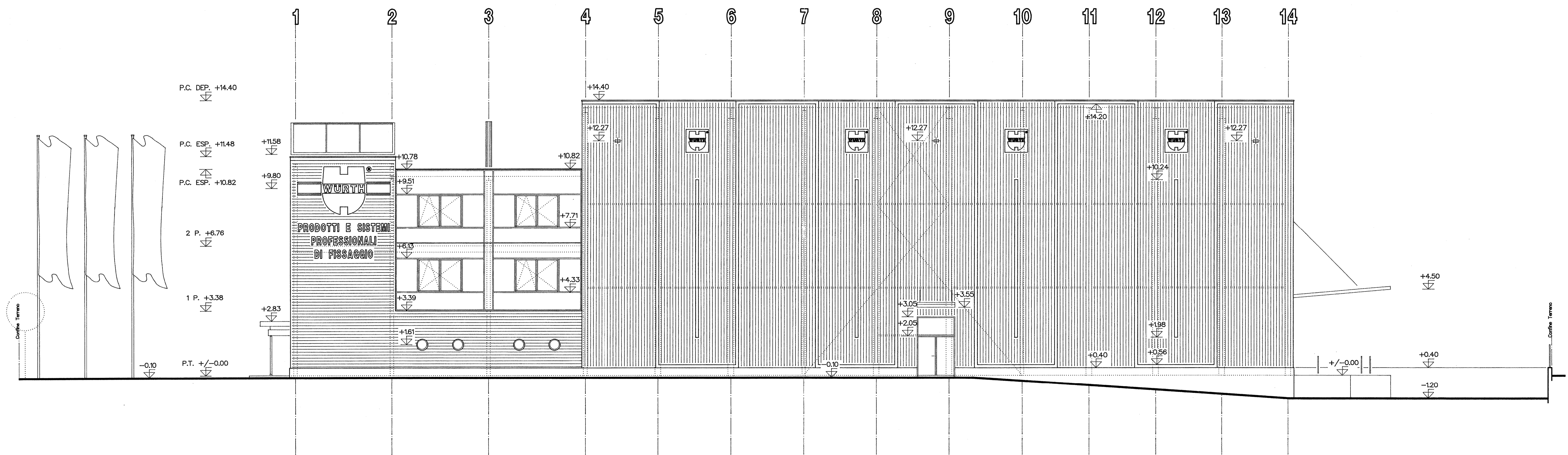
FACCIATA OVEST
